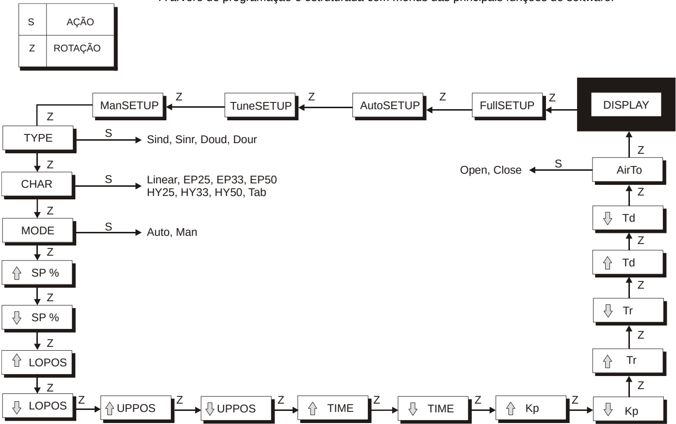
Figura 4.7 - Árvore de Programação Local
