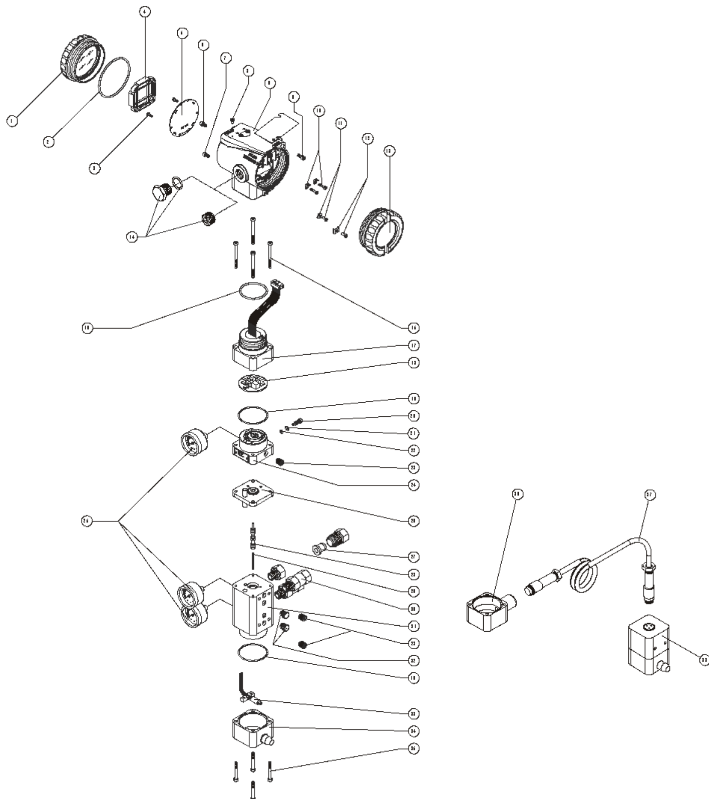
Figura 7.1 – Vista Explodida
