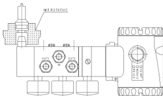
Figura 1.2 – Posicionador e Ímã Rotativo
