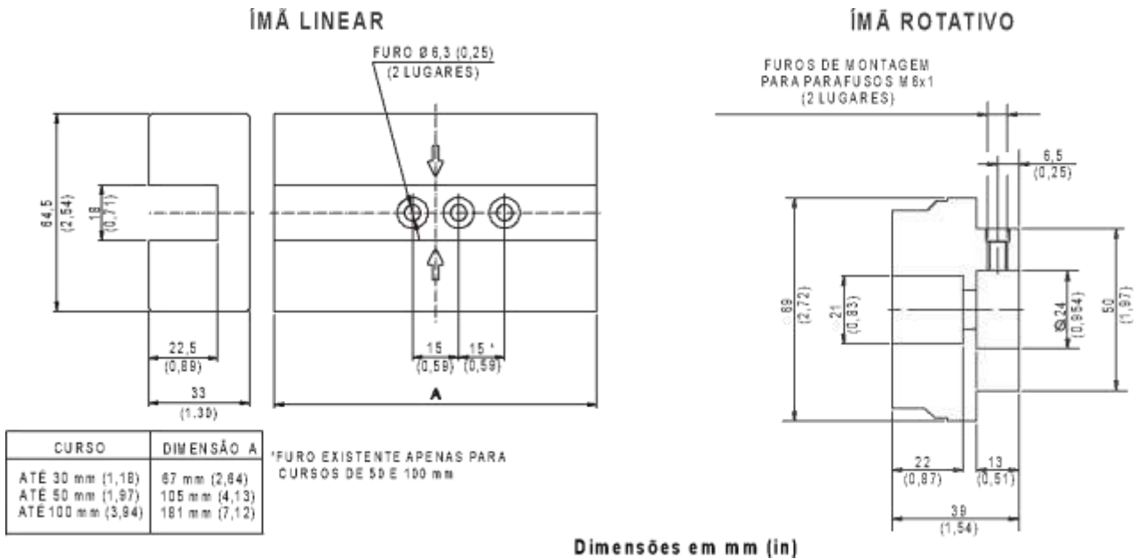
Figura 1.8 - Desenho Dimensional dos Ímãs
