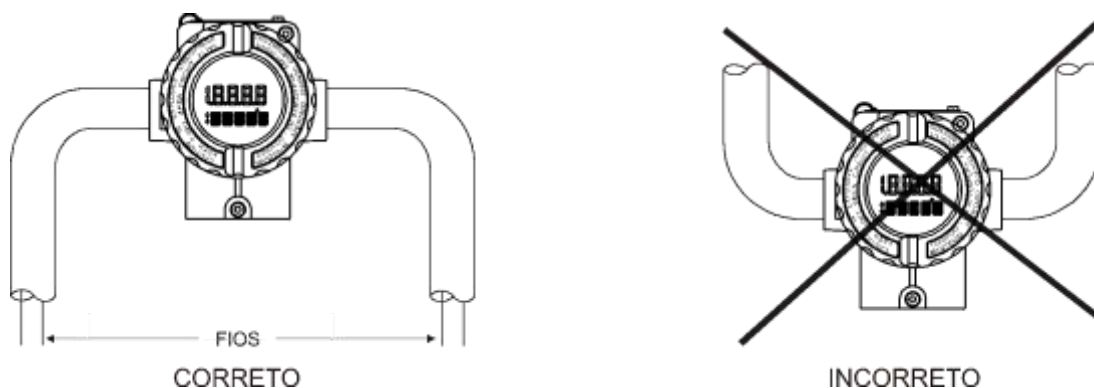
Figura 1.11-A – Diagrama de Instalação do Eletroduto
