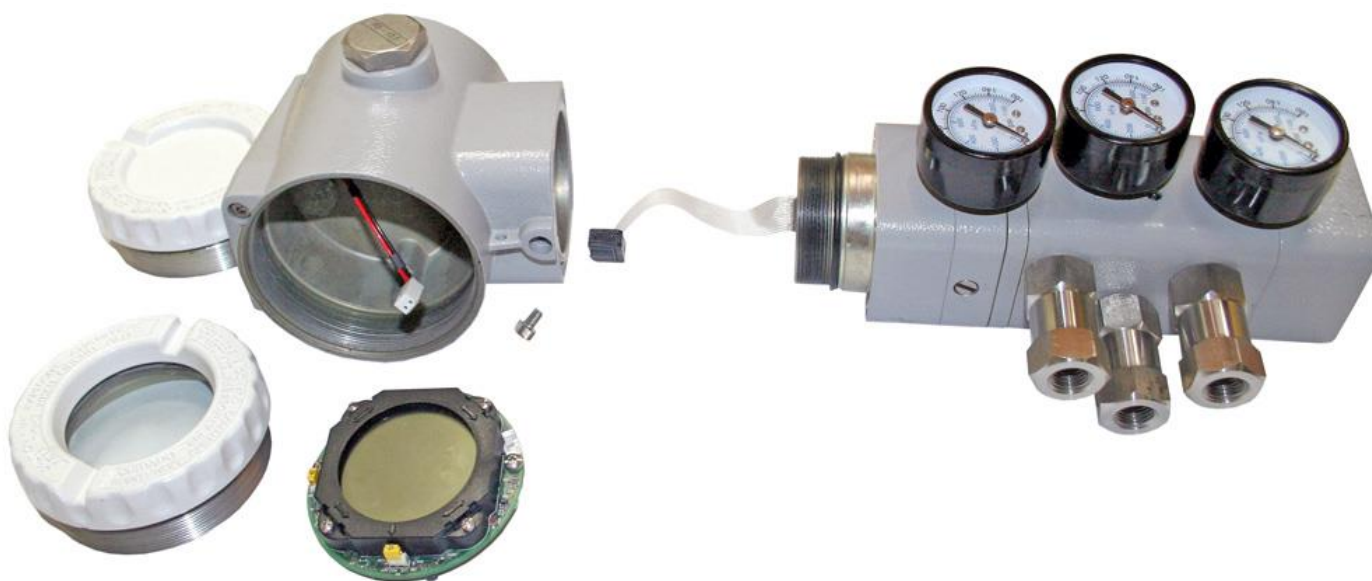
Figura 6.5 – Carcaça desmontada, separada do Transdutor
