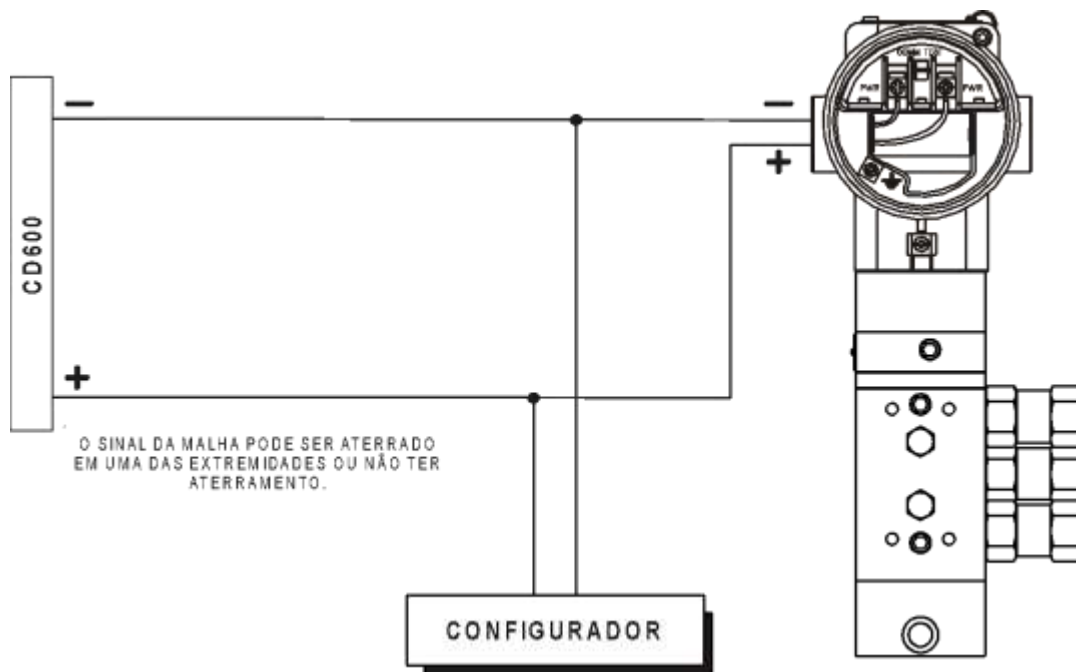
Figura 1.14 - Diagrama de Ligação do FY400 Hart, com o CD600
