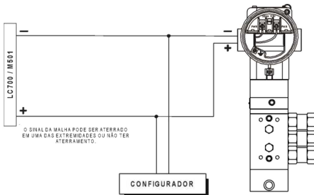
Figura 1.15- Diagrama de Ligação do FY400 Hart, com LC700/M501
