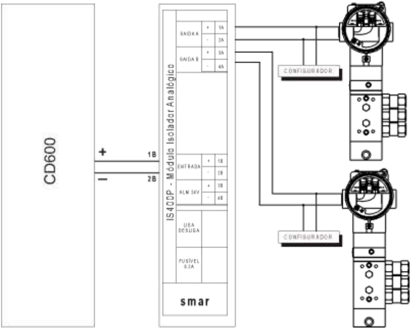
Figura 1.17 - Diagrama de Ligação dos Posicionadores, com CD600, em Split Range, em cartões com impedância máxima de saída menor 1100 \Lambda
