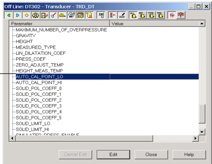
Figura 3.10 - Autocalibração Inferior de Concentração/ Densidade
