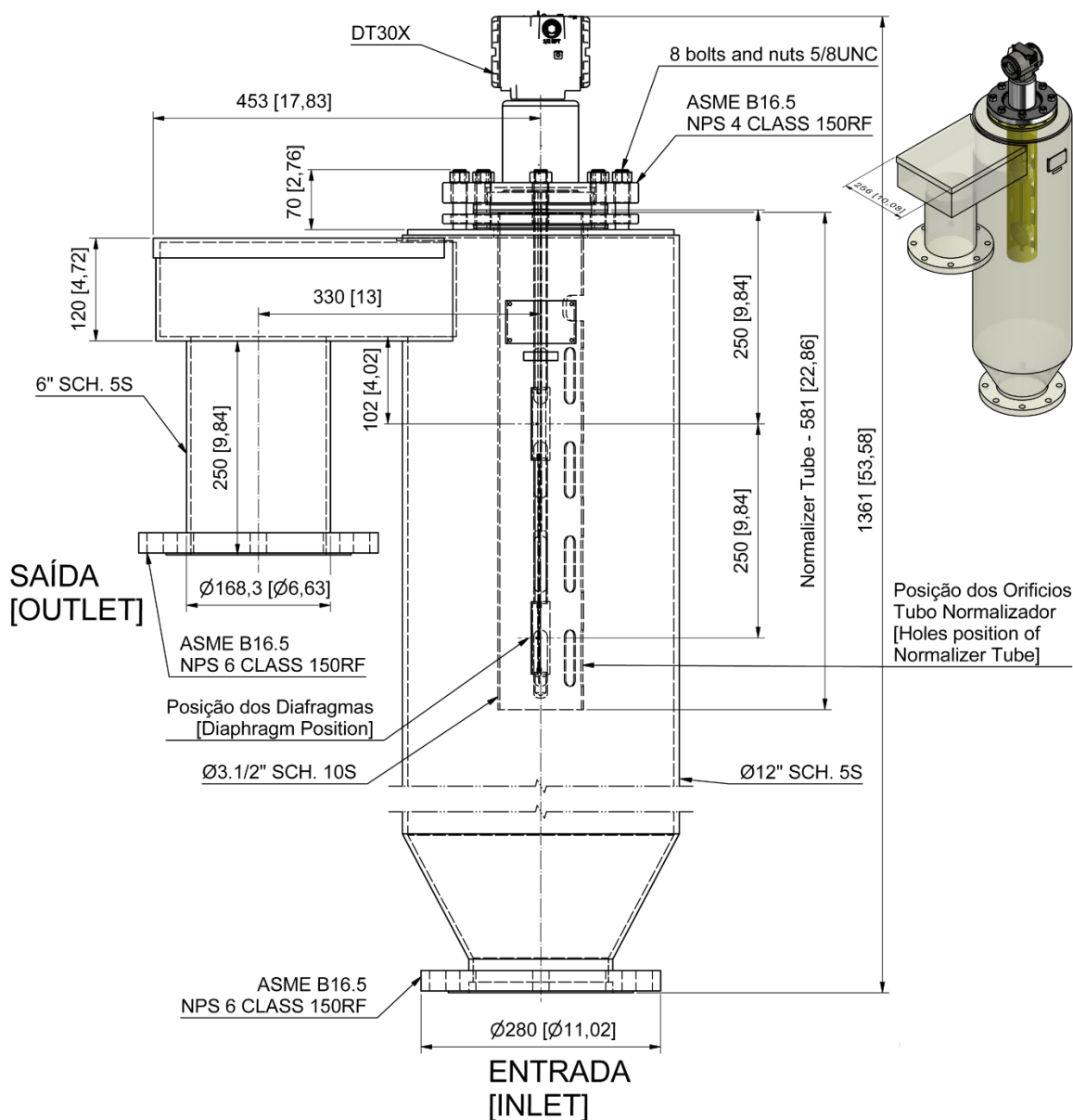
Figura 1.9 – Tipos de Instalação para o DT302 (C)
