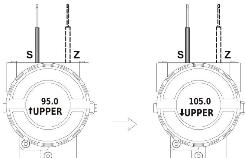
Figura 3.22 – Passo 5 – DT302
