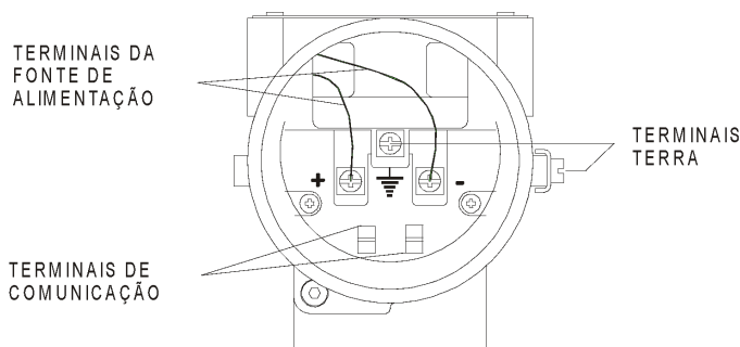
Figura 1.23 - Bloco Terminal
