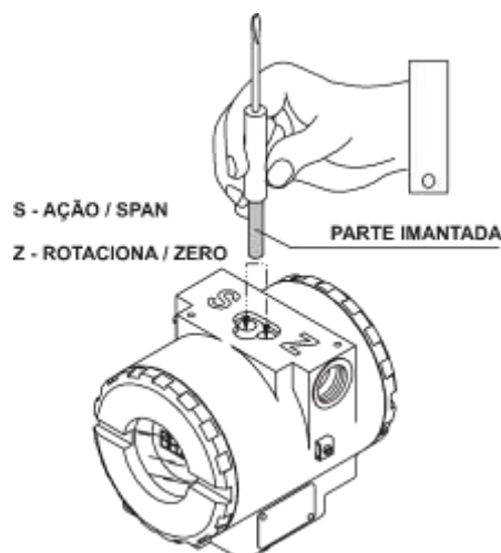
Figura 3.16- Orifícios do Ajuste Local
