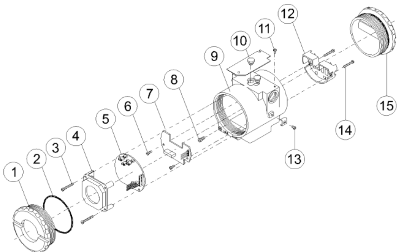
Figura 4.2 - Vista Explodida
