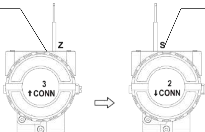
Figura 3.23 - Passo 6 - TT302
