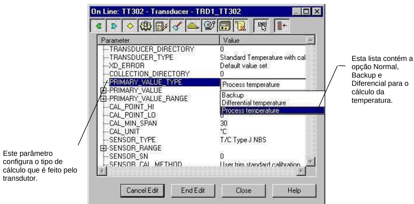
Figura 3.4 - Configuração do Tipo da Variável Primária
