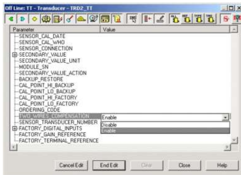
Figura 3.5 - Compensação da Resistência da Linha
