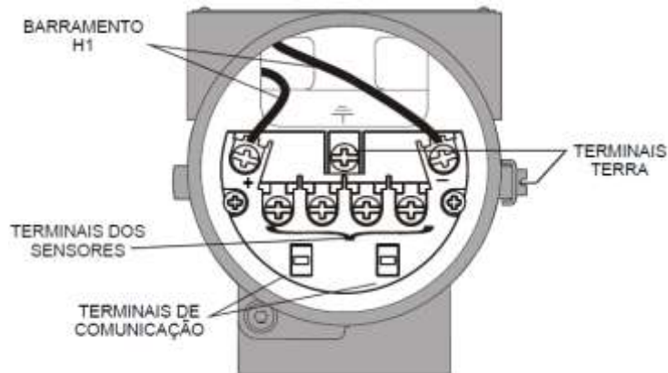
Figura 1.2 - Terminais Terra
