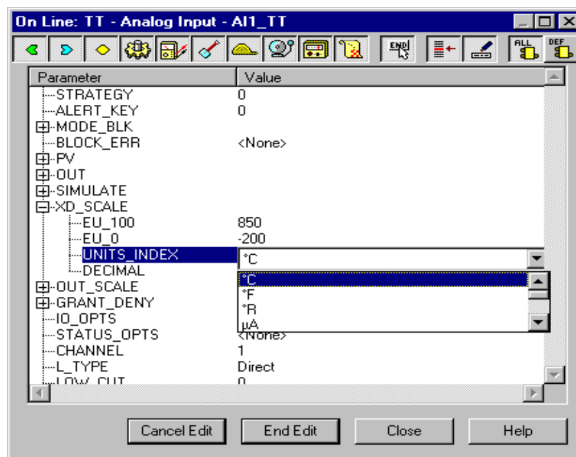
Figura 3.9 – Unidade do Sensor de Temperatura
