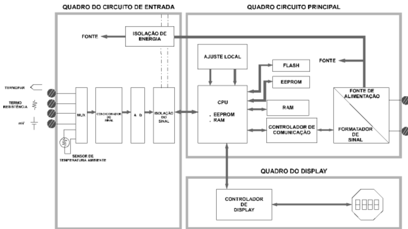
Figura 2.1 - Diagrama de Bloco do TT302
