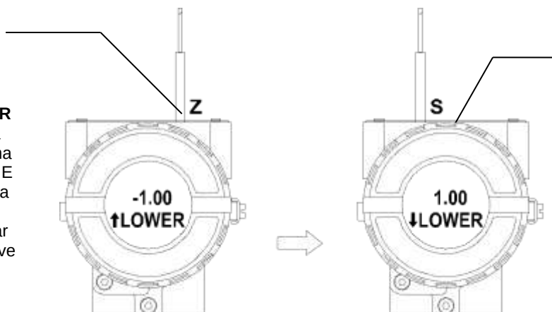
Figura 3.21 - Passo 4 - TT302
