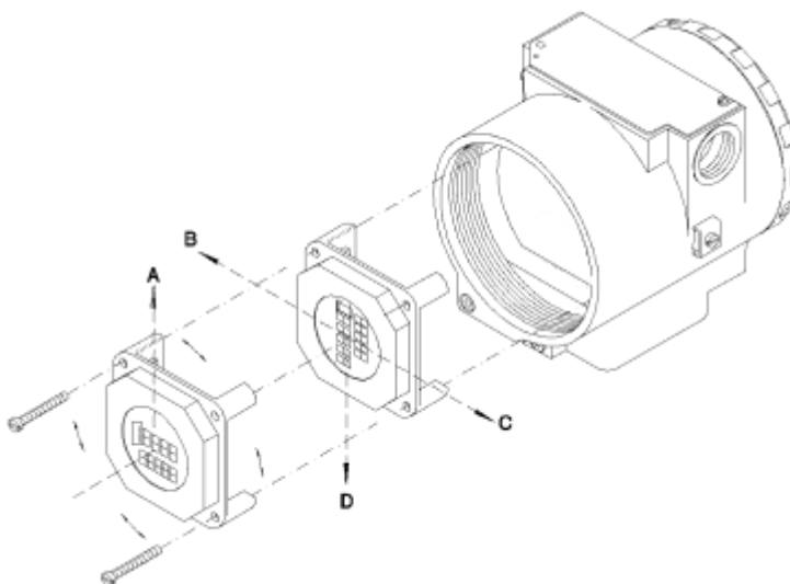
Figura 4.1 - Quatro Posições Possíveis para o Display
