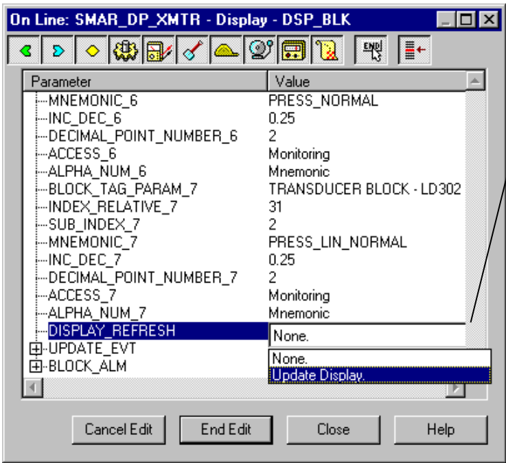
Figura 3.14 - Parâmetros para Configuração doe Ajuste Local
