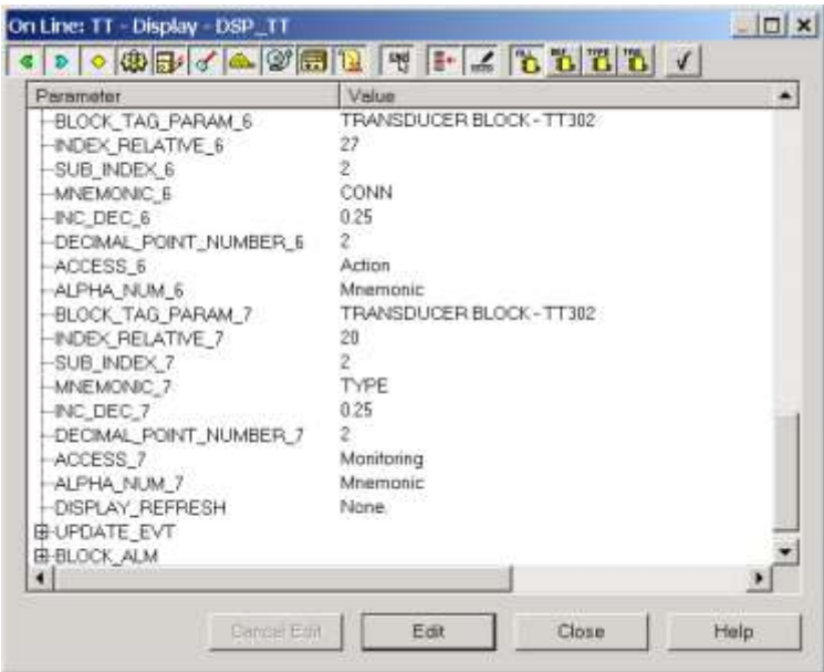
Figura 3.14 - Parâmetros para Configuração doe Ajuste Local
