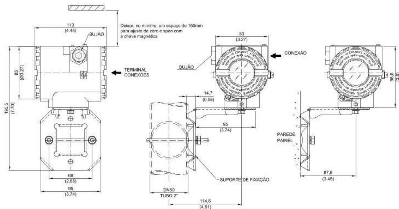
Figura 1.3 - Desenho Dimensional e Posições de Montagem
