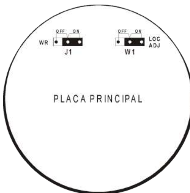
Figura 3.17- Jumpers J1 e W1
