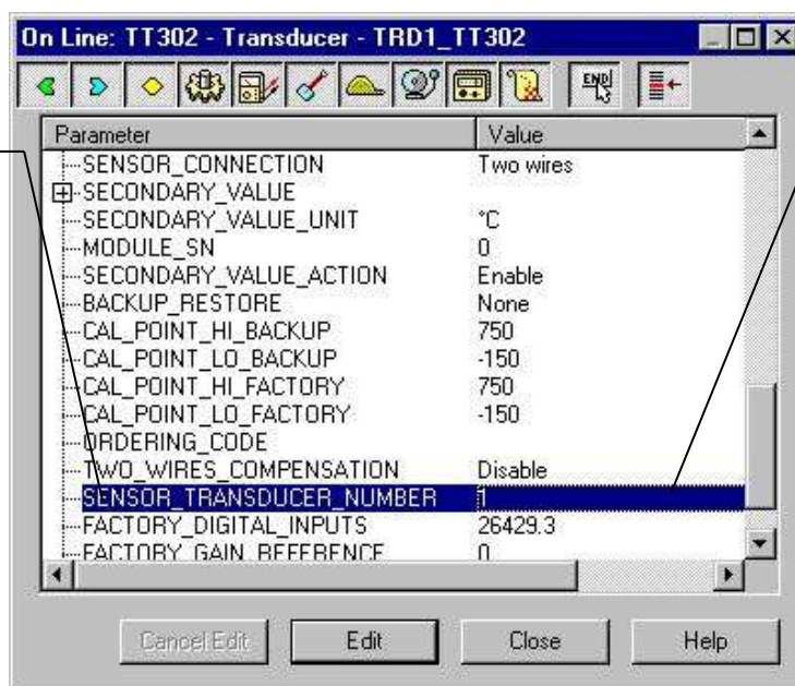
Figura 3.1 – Configuração do Numero do Transdutor
